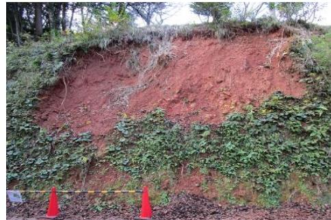
崩落した法面（近景）
