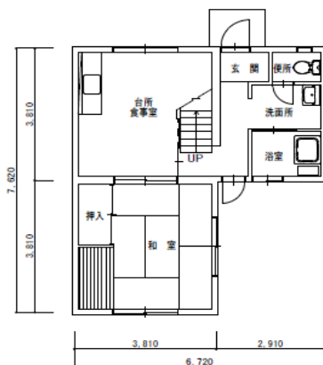
1階平面図
