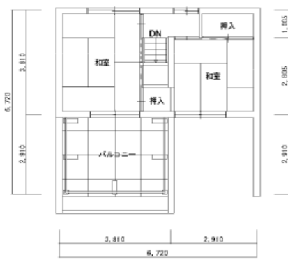
2階平面図
