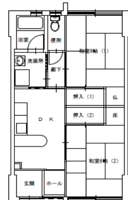
1階平面図
