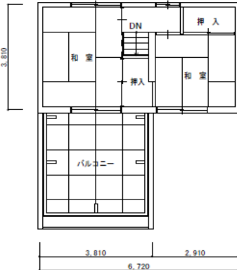
2階平面図
