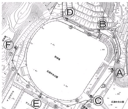
ナイター照明塔配置図
