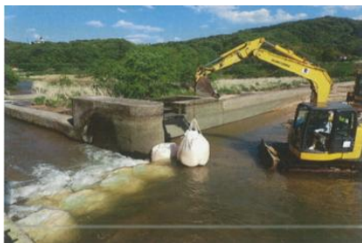
富田頭首工取水口緊急仮設工事
