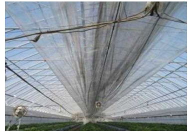
いちごハウス内張(上面)開閉装置
