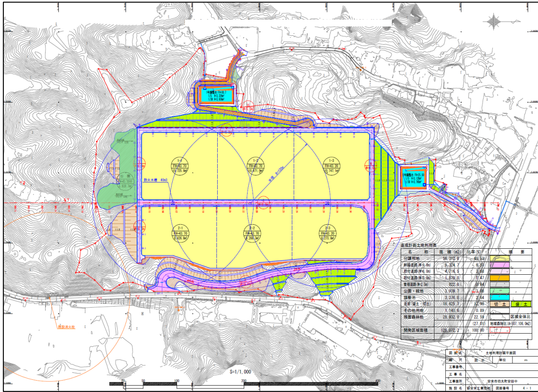
新安来工業団地(仮称)整備事業 計画平面図
