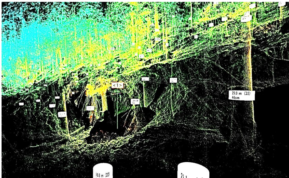
3次元計測システムによる解析図(材積等の資源量の把握、作業道の設計等に活用)
