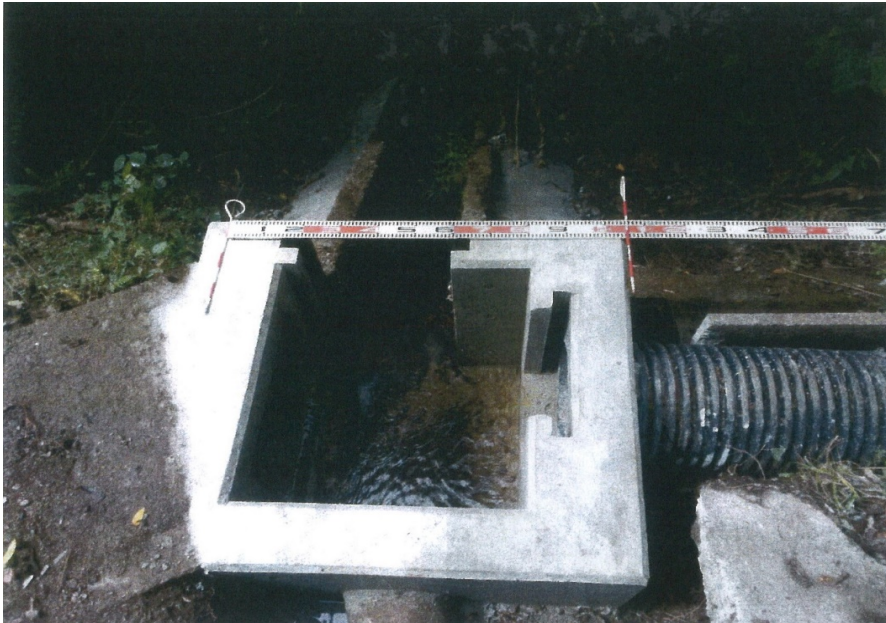
集水枡工
