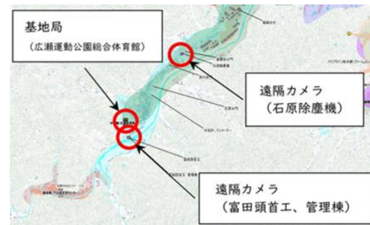
通信基地局 1基、遠方監視カメラ 2箇所
