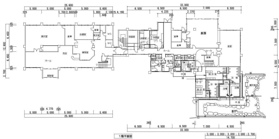
19-2 平面図 (1階)
