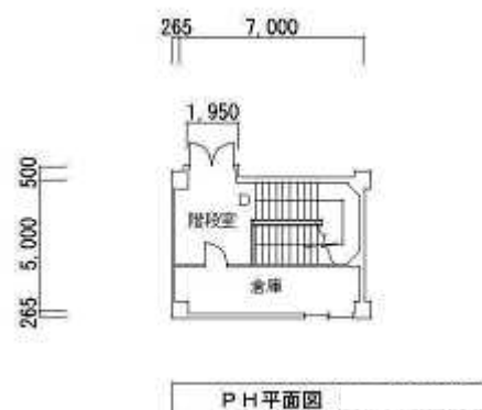
19-4 平面図 (PH)
