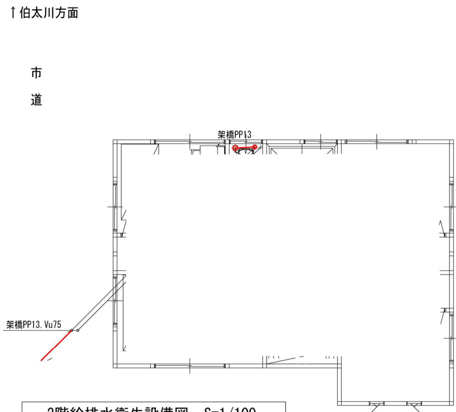
2階給排水衛生設備図 S=1/100
