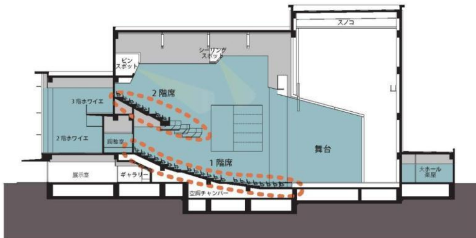
大ホール断面図
