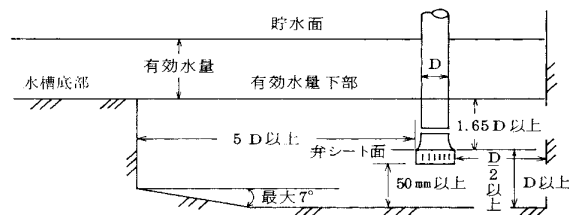
(イ) サクシヨンピットを設ける場合
