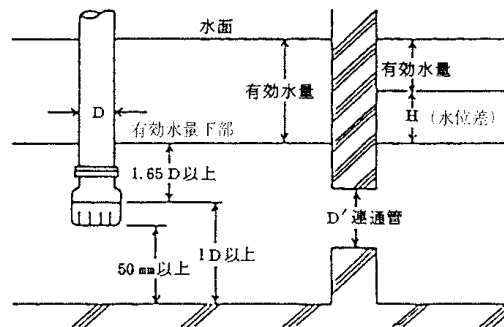
(イ) サクシヨンピットを設ける場合
