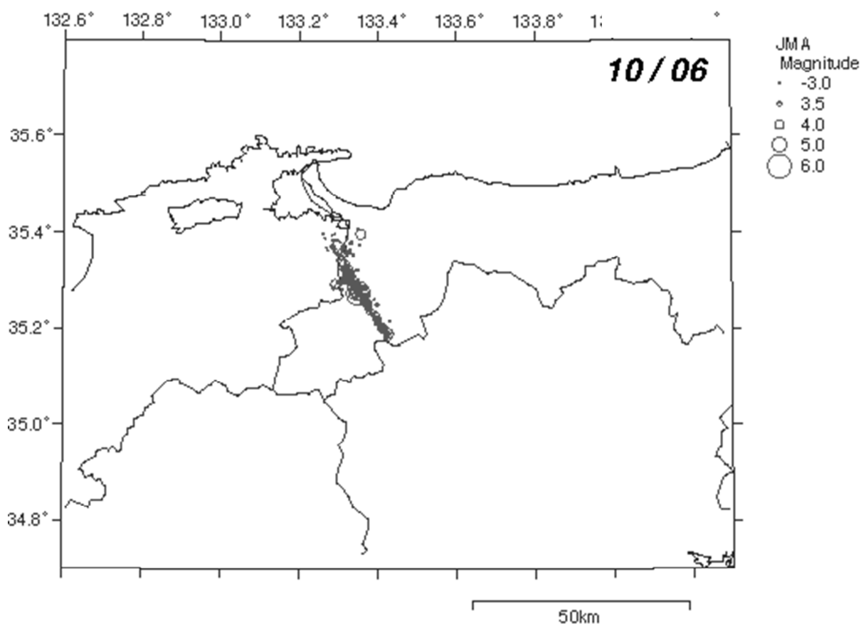
平成12年10月6日の震源分布（地震調査研究推進本部）
