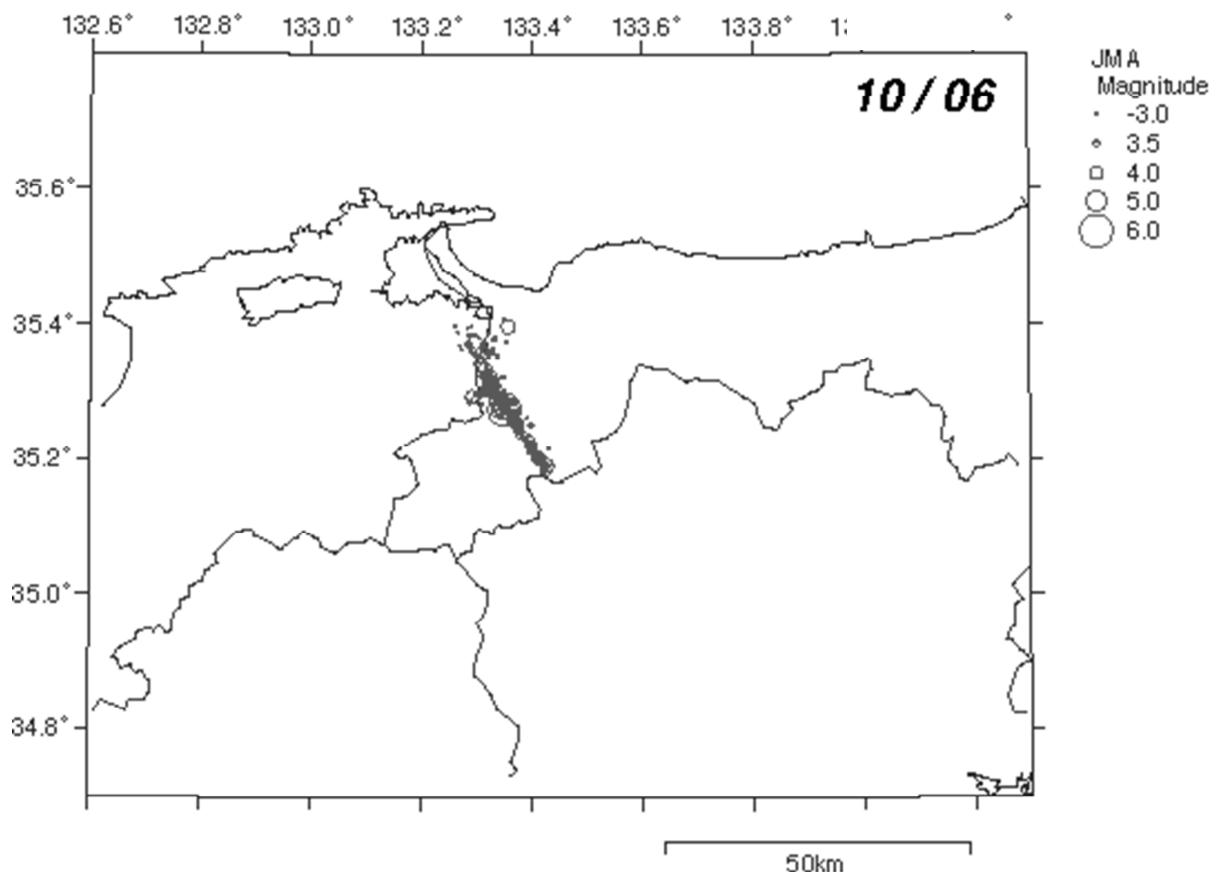
平成１２年１０月６日の震源分布（地震調査研究推進本部）
